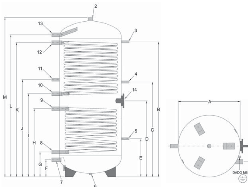
Rozměrový výkres se vztahuje k modelu UBHP 1000 DC
