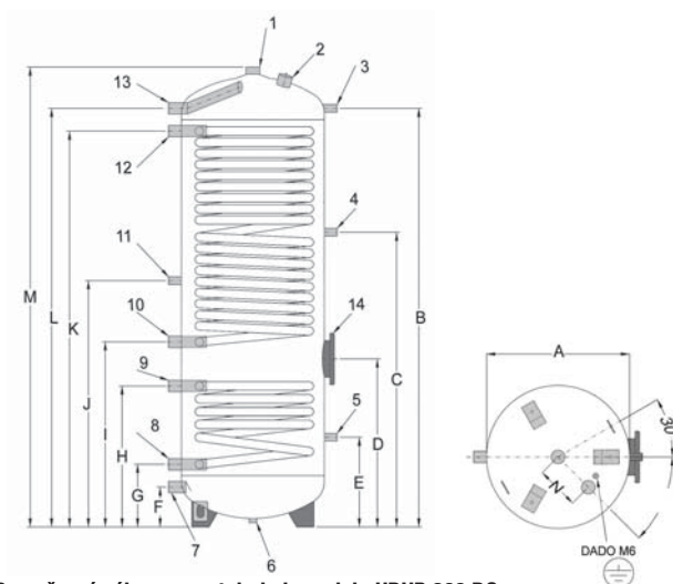
Rozměrový výkres se vztahuje k modelu UBHP 300 DC
