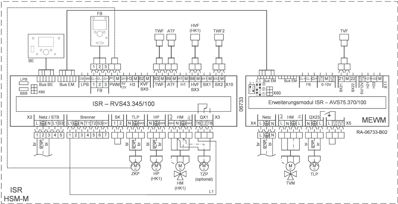
Obr.9 Schéma zapojení
