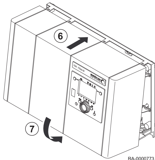
Obr.12 Zavření skříně
