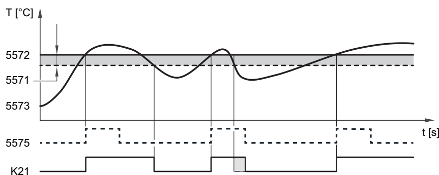
Obr.28 Sledování nadměrné teploty
