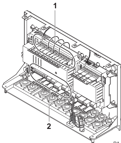
Obr. 14 Vedení kabelů uvnitř skříně
