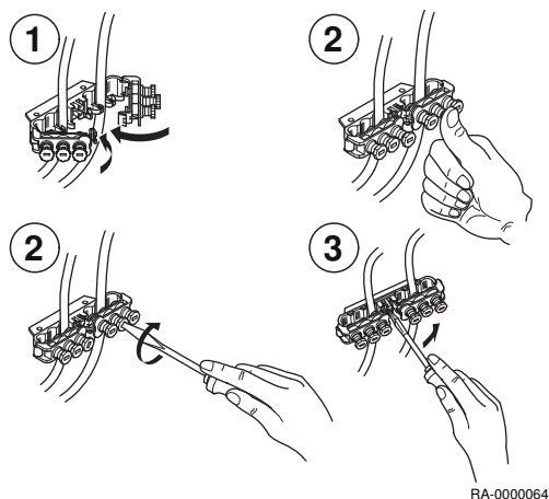
Obr.13 Odlehčení tahu
