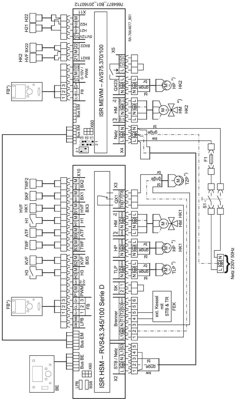
Obr.2 Schéma zapojení
