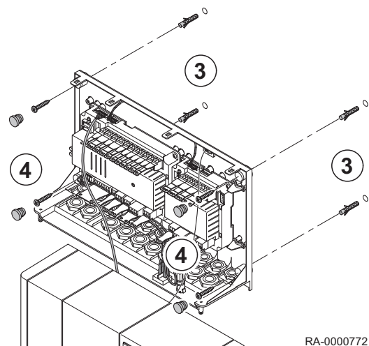
Obr.12 Zavření skříně
