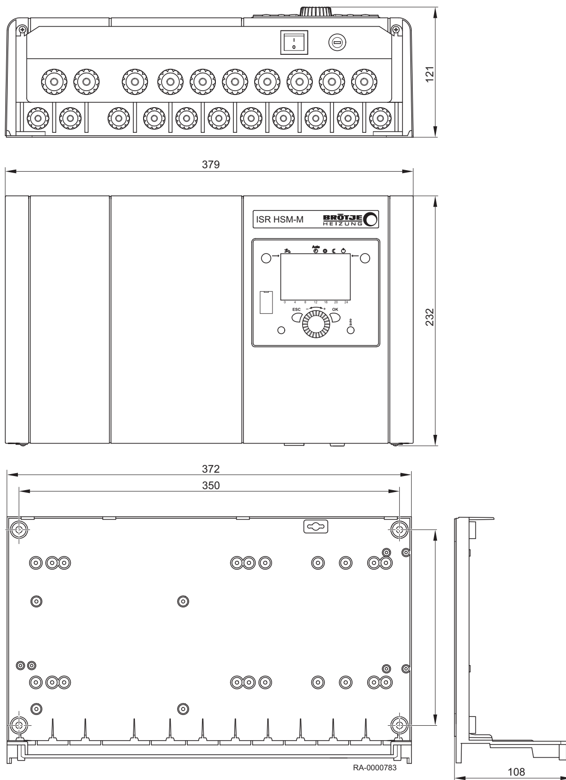
Obr.1 Rozměry
