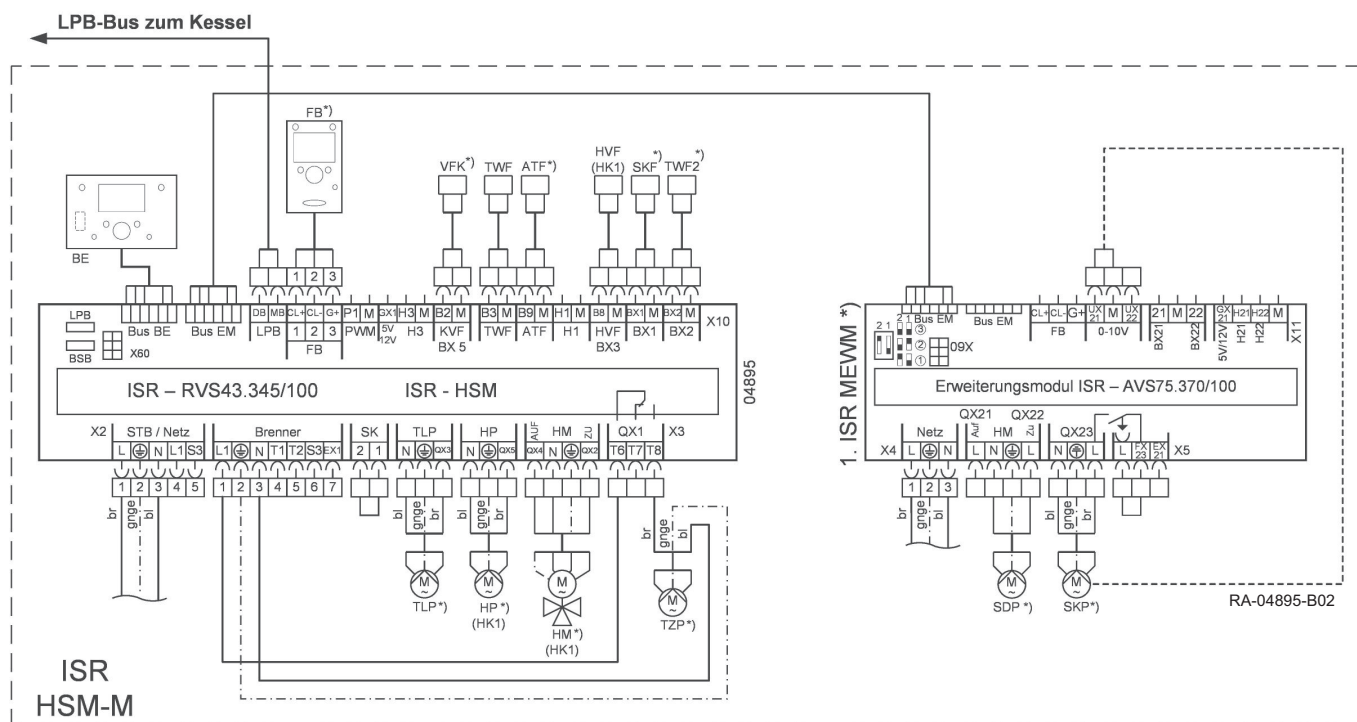
Obr.7 Schéma zapojení
