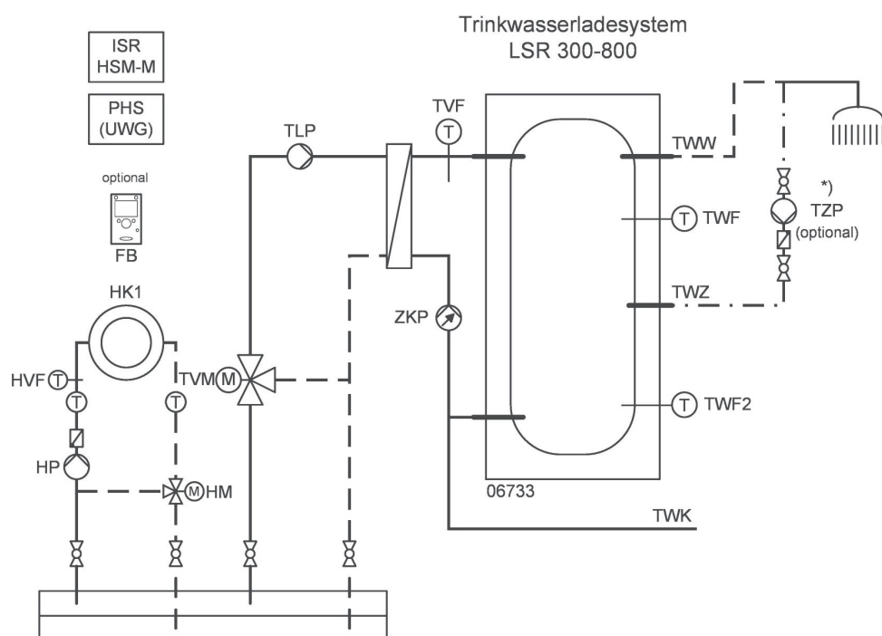
Obr.8 Příklad 2 aplikace: Topný okruh směšovače s pokojovým zařízením a ohřivačem užitkové vody – schéma hydraulického okruhu
