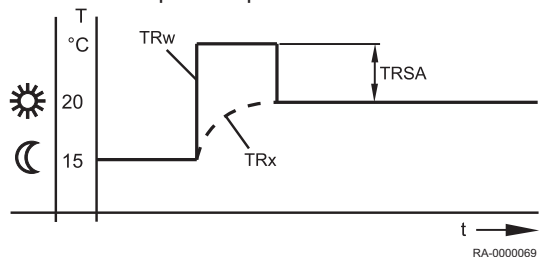
Obr. 19 Podpůrné topení
