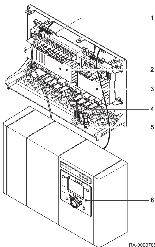
Obr.3 Přehled HSM-M
