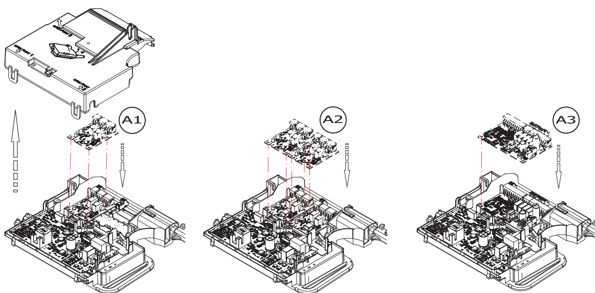
Obr.134 Umiestnenie a upevnenie dosiek príslušenstva v kotle
