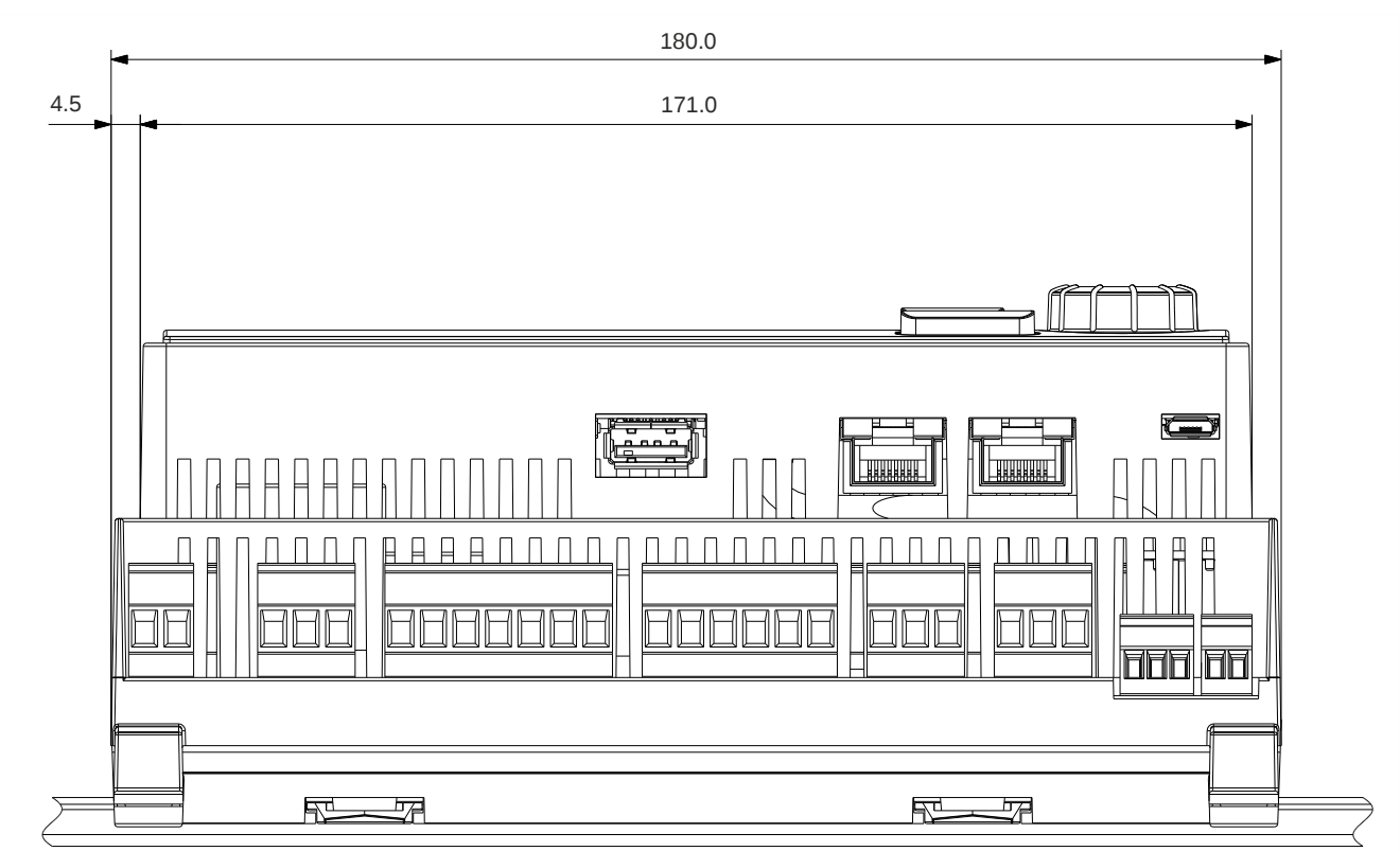
Pohled zdola
