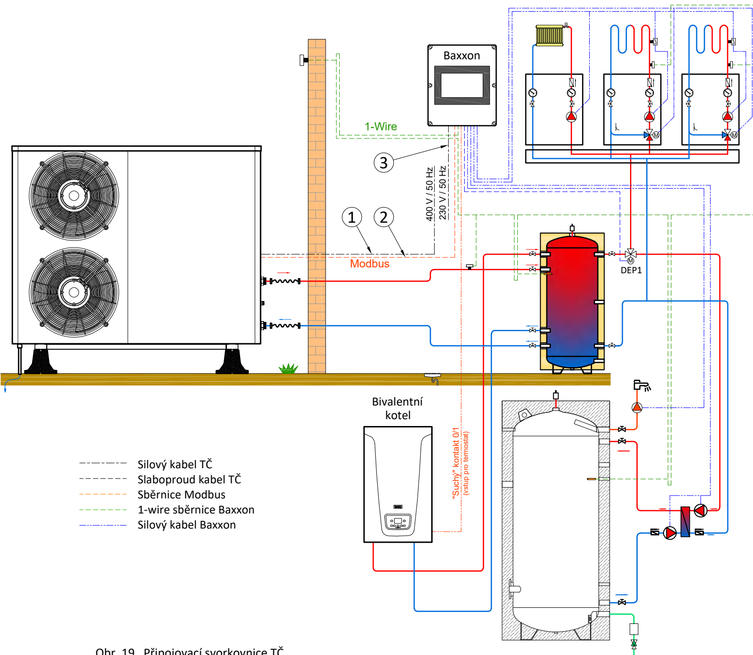
Obr. 19 Připojovací svorkovnice TČ
